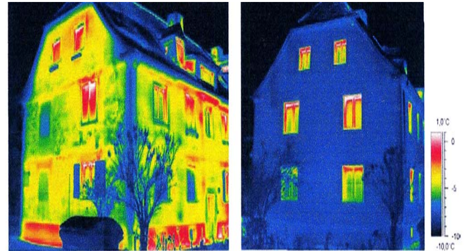
Thermografie vor Sanierung
