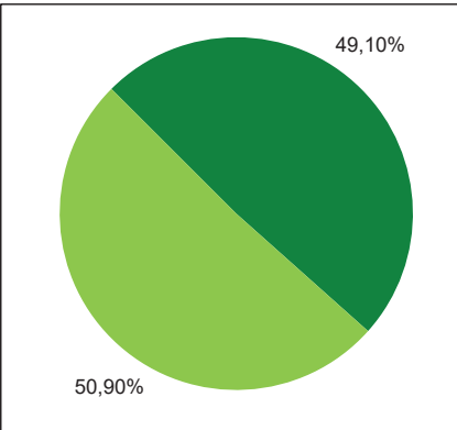
Produktmix E-Ladesäulen
