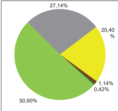
Verbleibender Energieträgermix
